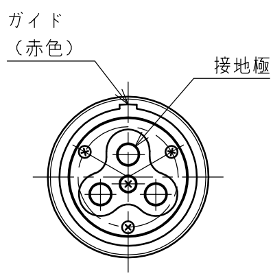
矢視 A - A
