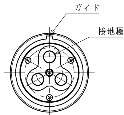
矢視 A - A
