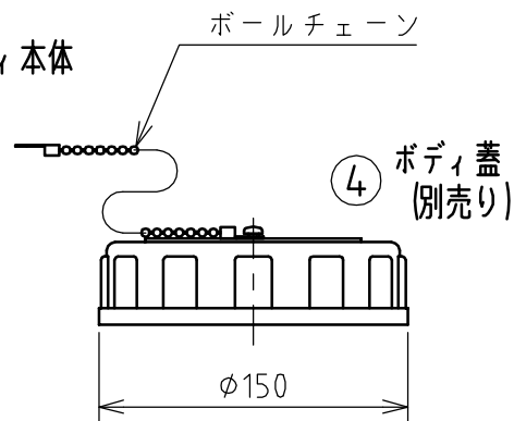
矢視 A - A
